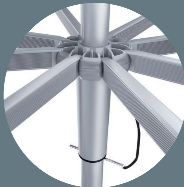
MOVIMENTO DI APERTURA E CHIUSURA A SPINTA PUSH OPENING AND CLOSING MOVEMENT
